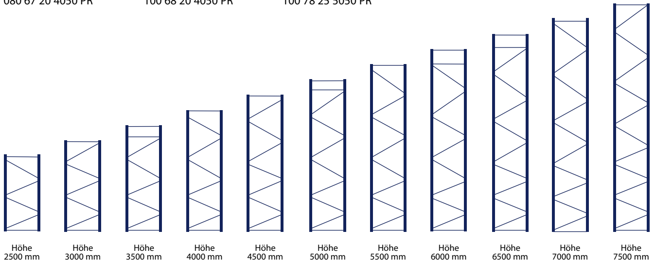
Ständertyp 080 67 20 4050 PR
